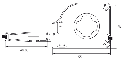
Cajón de mosquitero con tela y terminal
